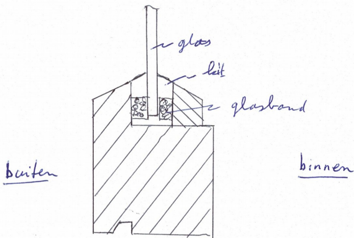
DOORSNEDE RAAM
